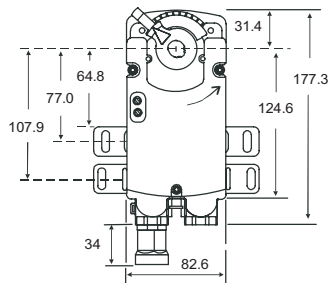
尺寸 (mm)
